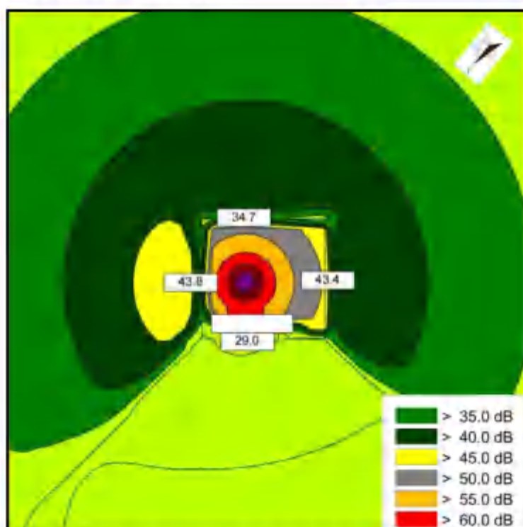
图 4-3 白洋 110kV 变电站现有#1 主变等声值线图
