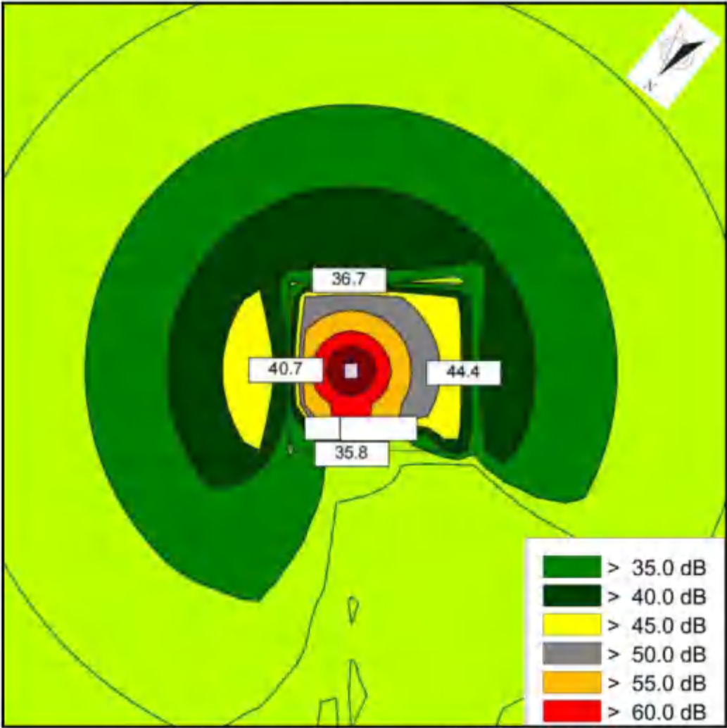
图 4-4 白洋 110kV 变电站本期#1 主变增容后等声值线图 (围墙外 1m, 距地面 1.2m)
