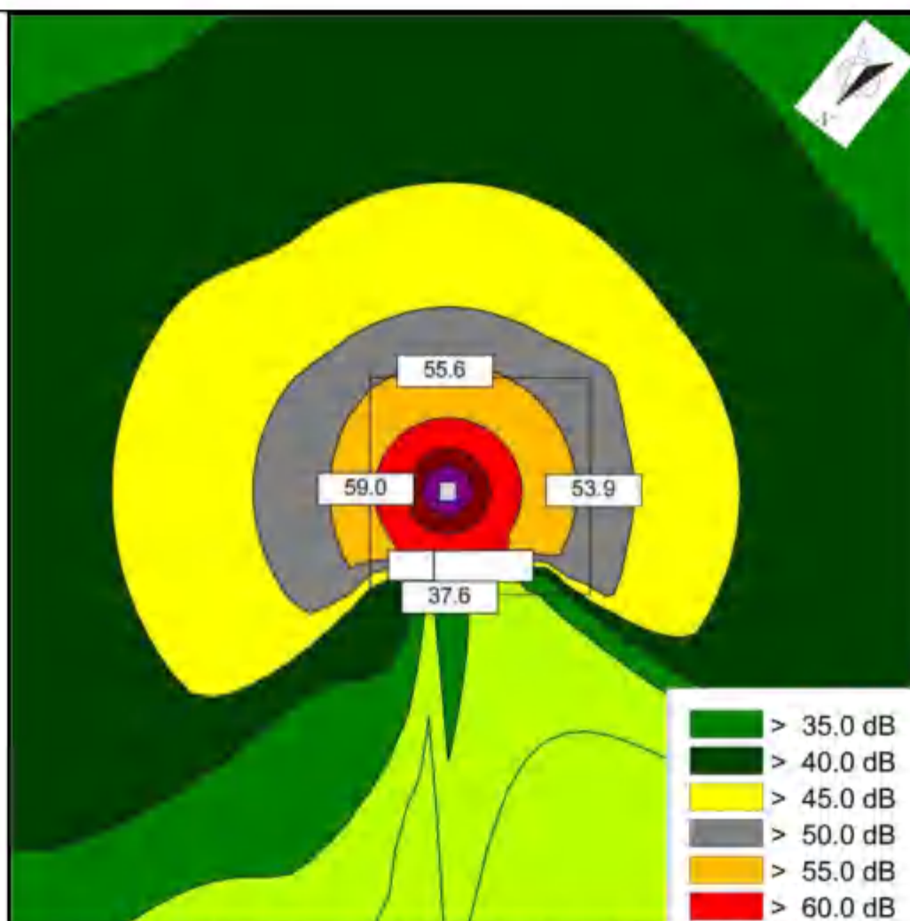
图 4-5 白洋 110kV 变电站本期#1 主变增容后等声值线图 (围墙外 1m, 围墙上方 0.5m)
