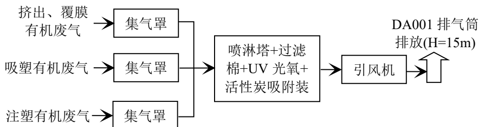
图 4.2-1 项目有机废气处理工艺流程图
