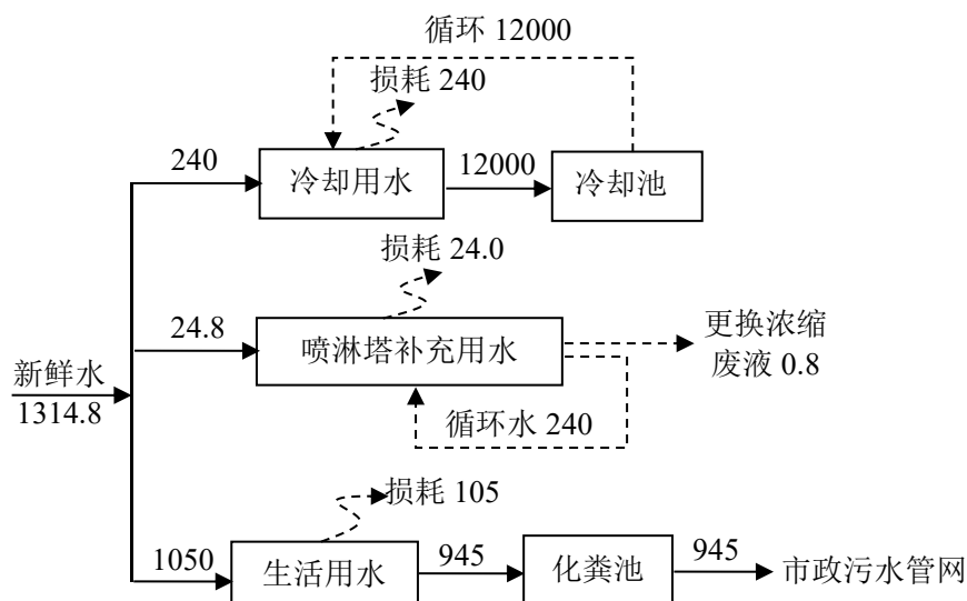
图 2.2-2 项目工程水平衡图 单位：m³/a
