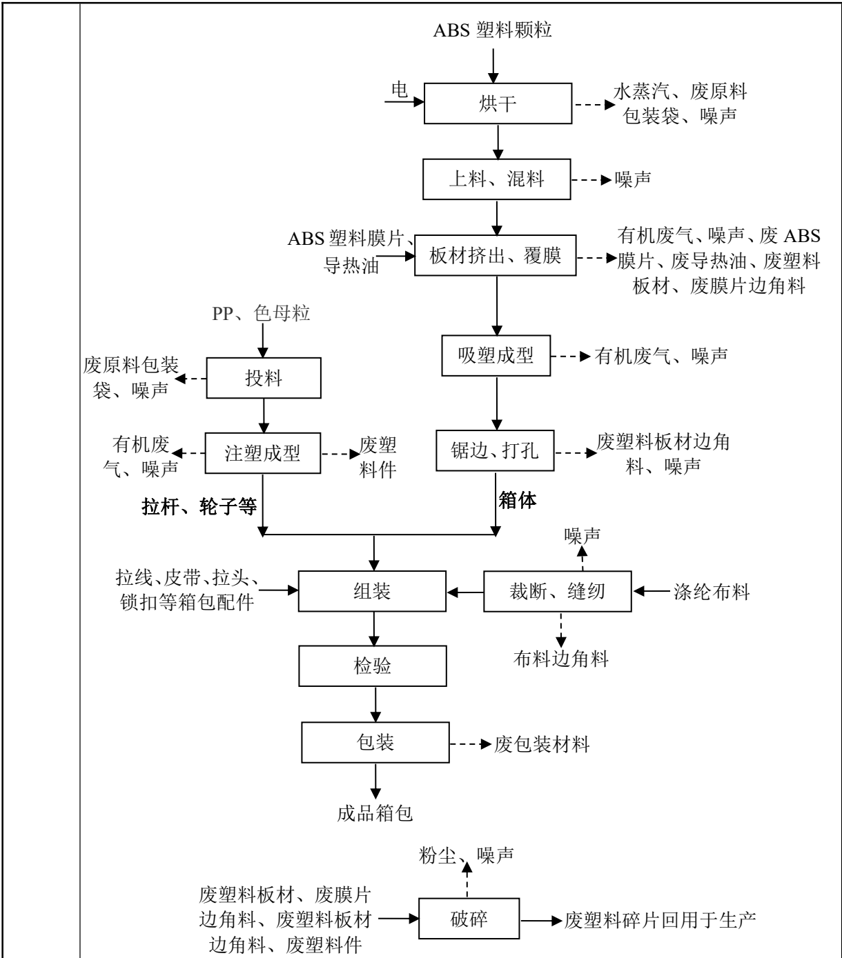
图 2.3-1 项目生产工艺流程及产污环节示意图
